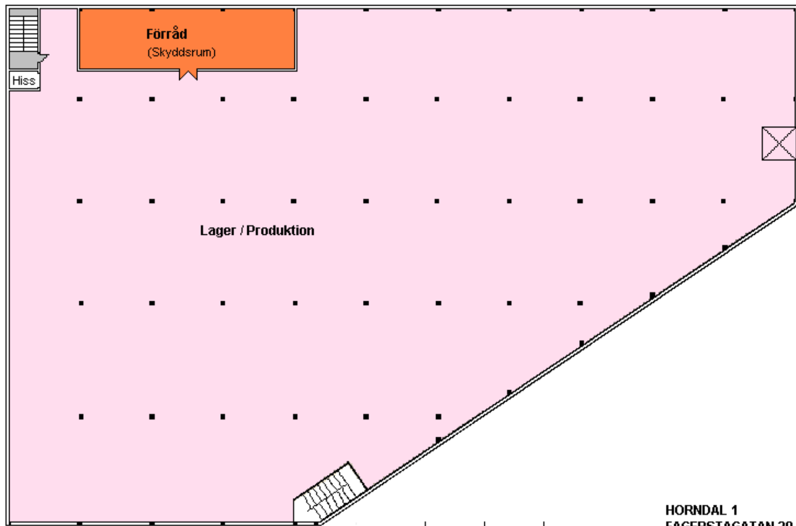
SUTERRÄNGVÅNING (-1 tr)
